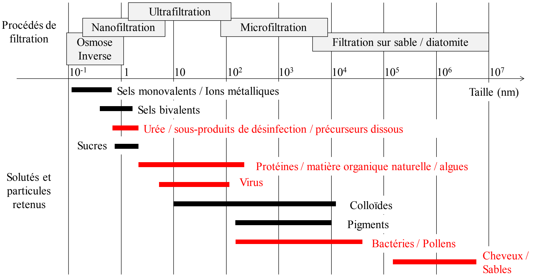
Positionnement des procédés de filtration en fonction du diamètre de pores membranaires et des molécules et particules à retenir
